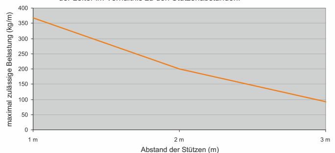
Der Graf zeigt die maximal zulässige gleichmäßige Belastung der Leiter im Verhältnis zu den Stützenabständen.
